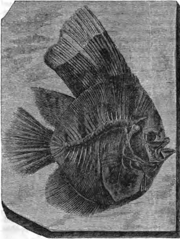
PLATAX ALTISSIMUS. A Ctenoid of Monte-Bolca. ( Eocene. )
